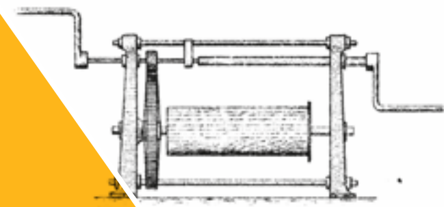
Ἐλατορῶλον χειροκίνητον
